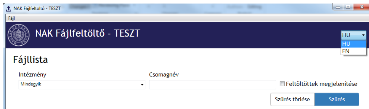
34. ábra: Nyelvválasztó
